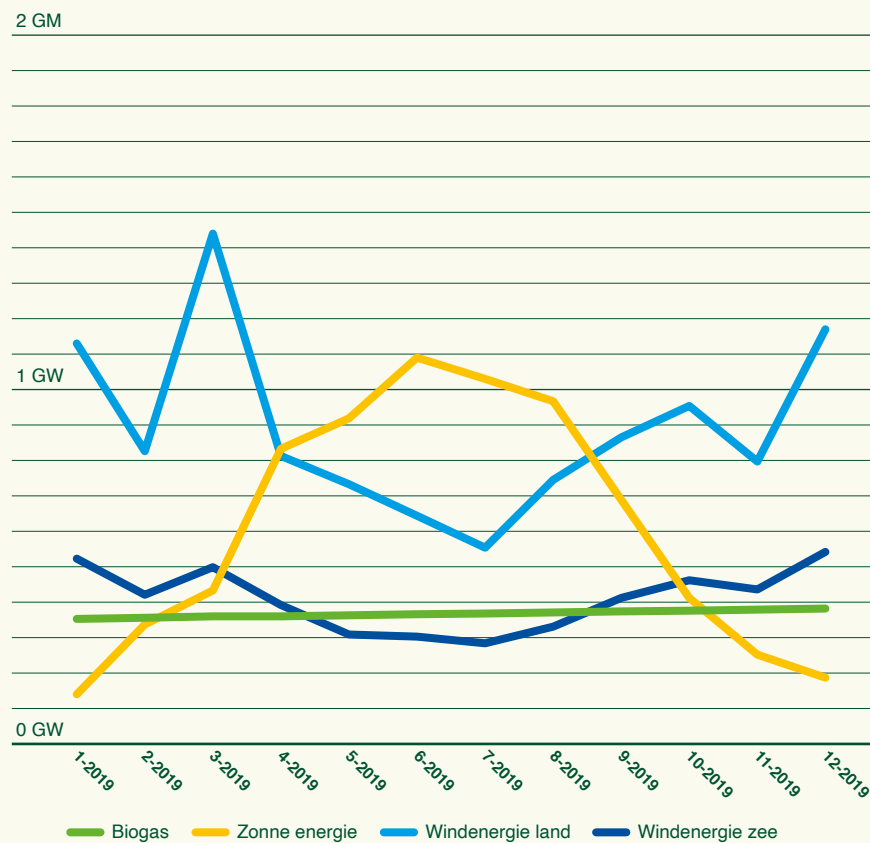
Energieproductie (GW/jaar)
